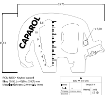
Technische Zeichnung
